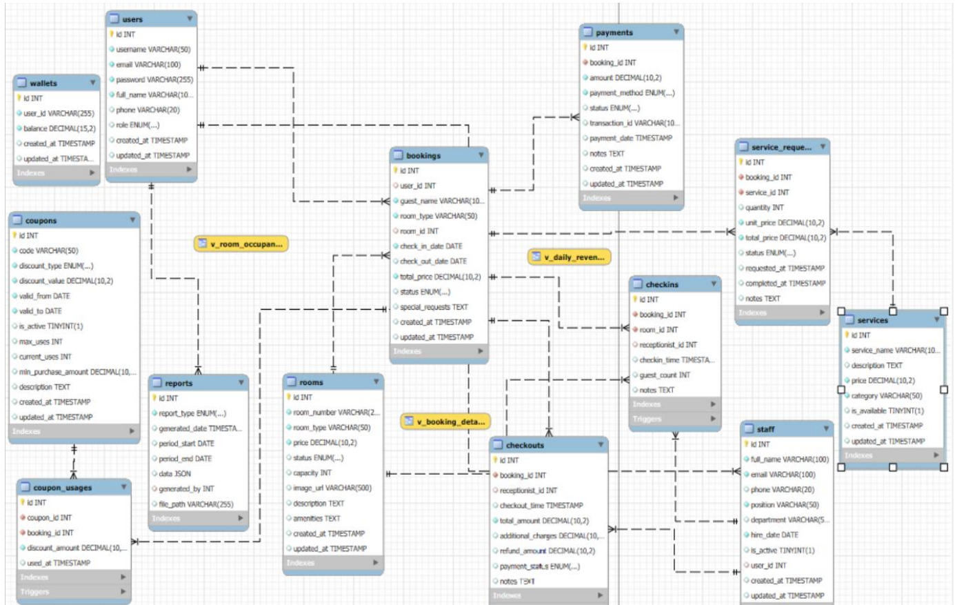
Figure 8: ER Diagram
